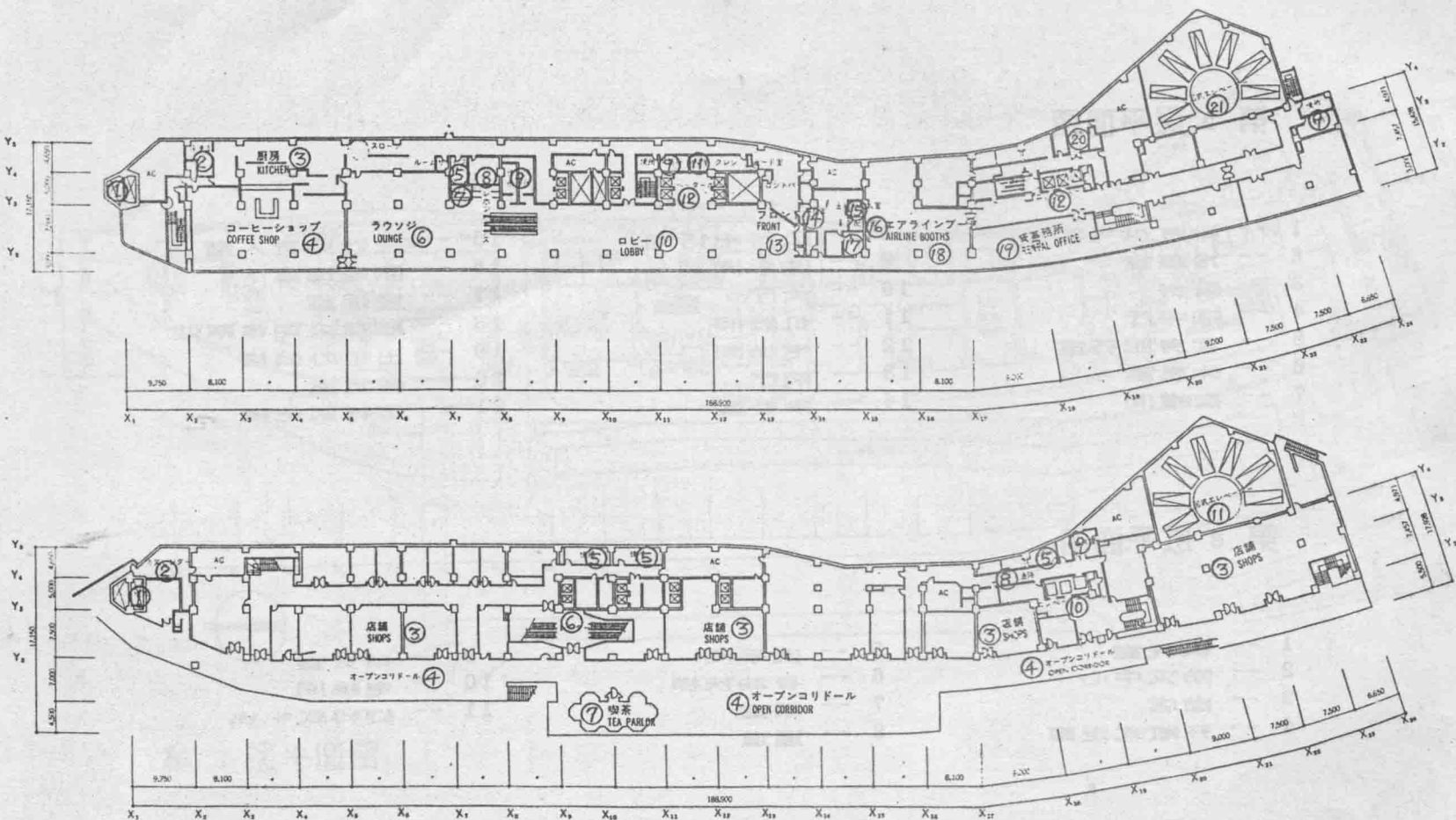
第 2、3 层平面图
