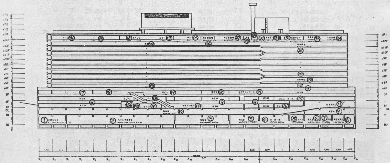
剖面图
