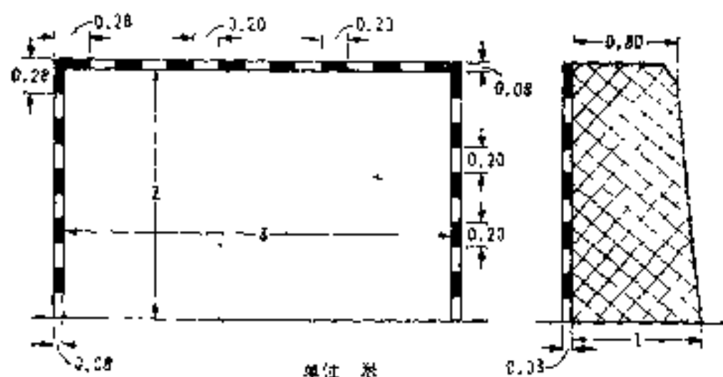
图二 球门和球门网
