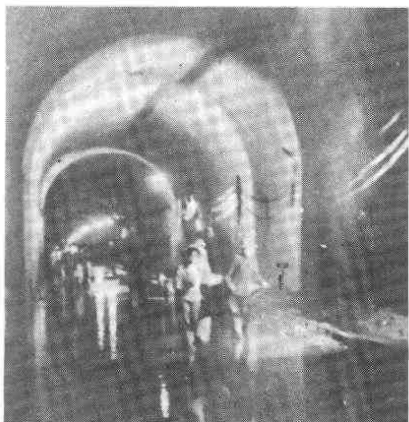
竣工后的清泉沟隧洞
