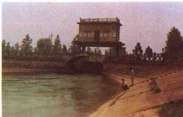
引丹工程总干渠的节制闸
