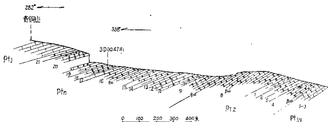
图6 宿县解集青铜山剖面图
