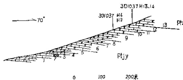
图5 濉溪县蚩顶山剖面图
