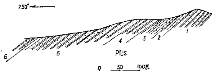
图4 泗县屏山剖面图
