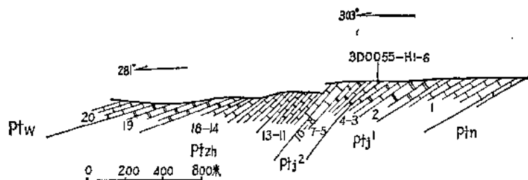
图 7 灵壁县陇山剖面图
