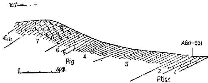
图 12 宿县褚蓝沟后剖面图
