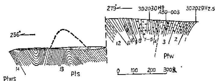
图9 宿县解集黑峰岭剖面图
