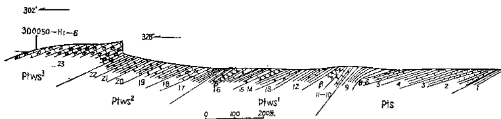
图10 宿县栏杆望山剖面图
