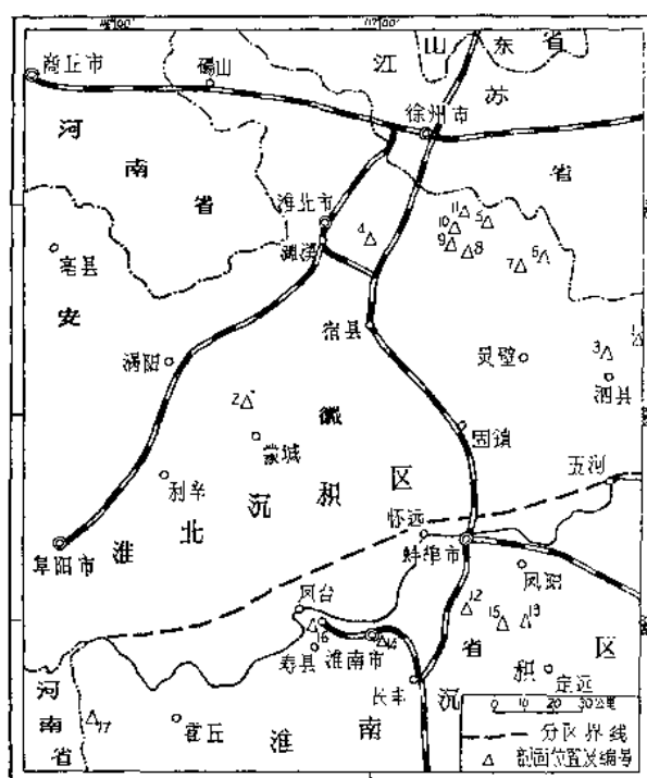
图1 皖北上前寒武系分区及剖面位置图
