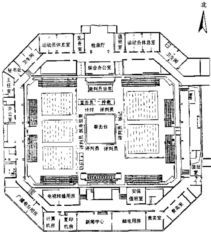
北京体育学院体育馆平面图
