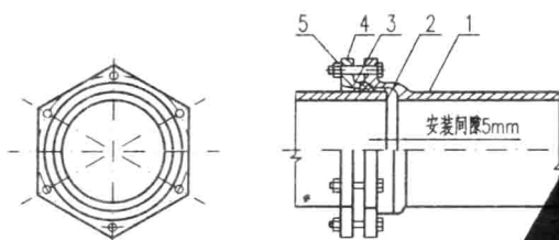
三耳接口型式
