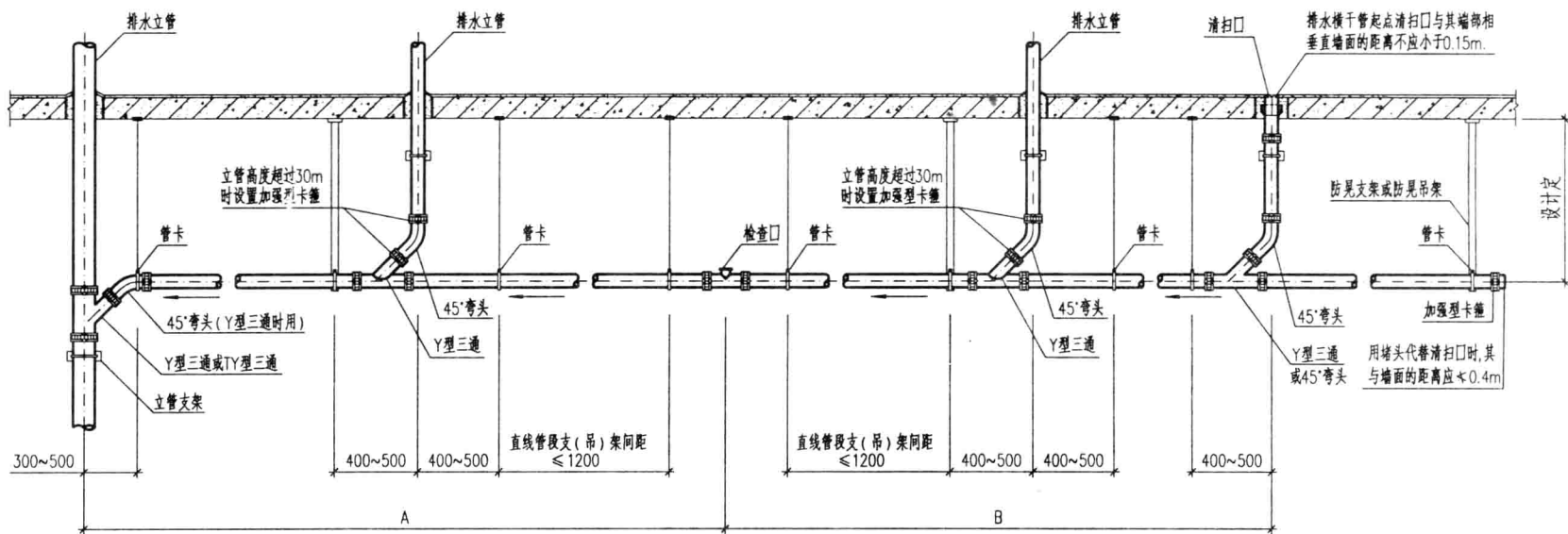
排水横干管的安装坡度及直线管段检查口或清扫口之间的最大距离
