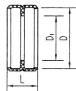
拉锁型橡胶密封圈
