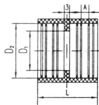
W型接口橡胶密封圈
