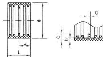
钢带型橡胶密封圈
