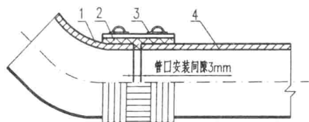
W型卡箍式接口型式 (DN50~300)
