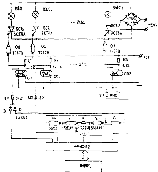
图4 交通灯驱动电路
