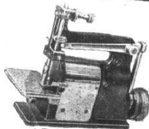
18型鎖邊縫紉機 供呢絨毛毯鎖邊用
