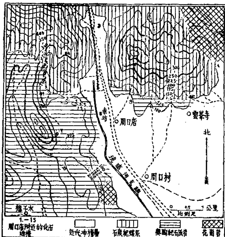
圖2 周口店附近地質圖
