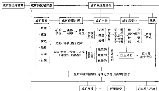
图1 成矿系统结构及其演化
