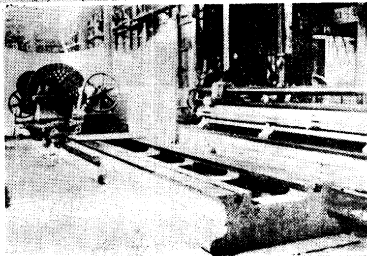
车炮箍车床
