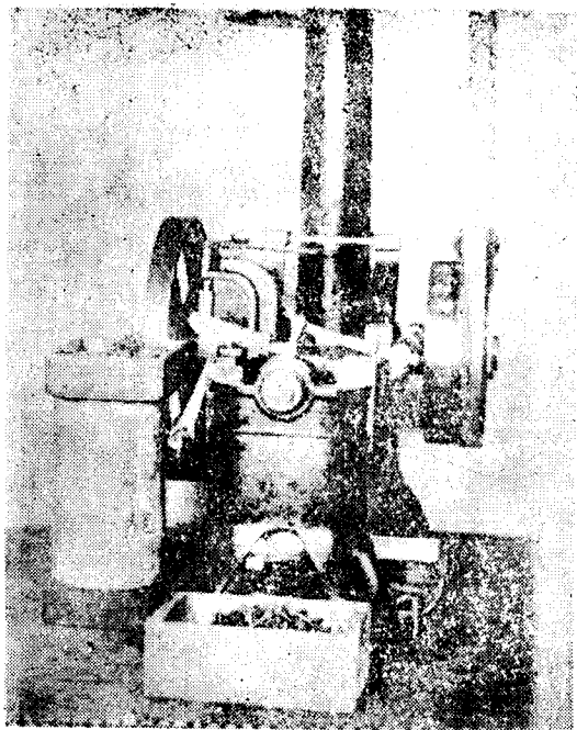
弹壳收口机
