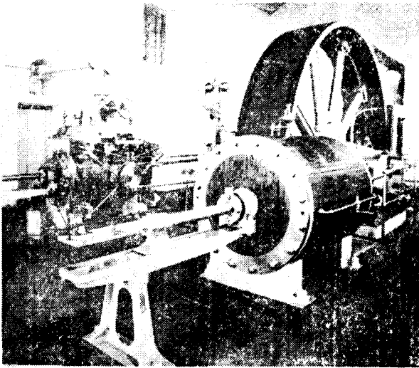
炮厂八十马力总引擎
