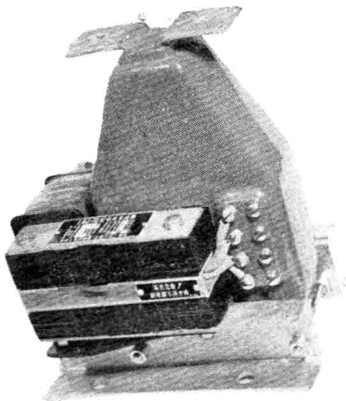
LQJ -- 15 高压电流互感器
