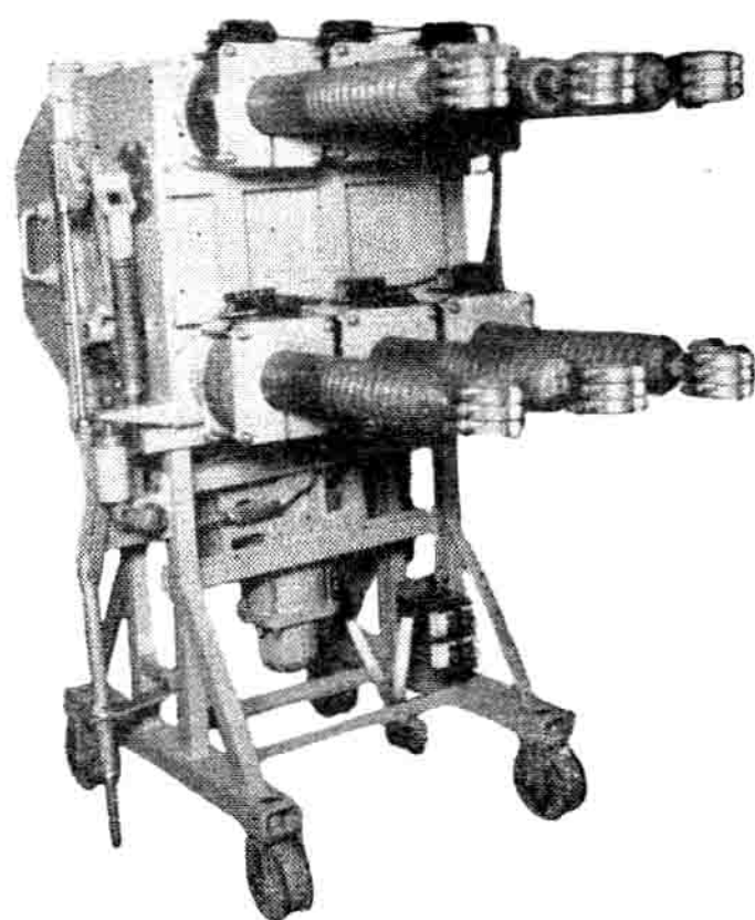
LN1-35 高压六氟化硫断路器
