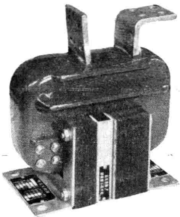
LZCJ—10 高压电流互感器
