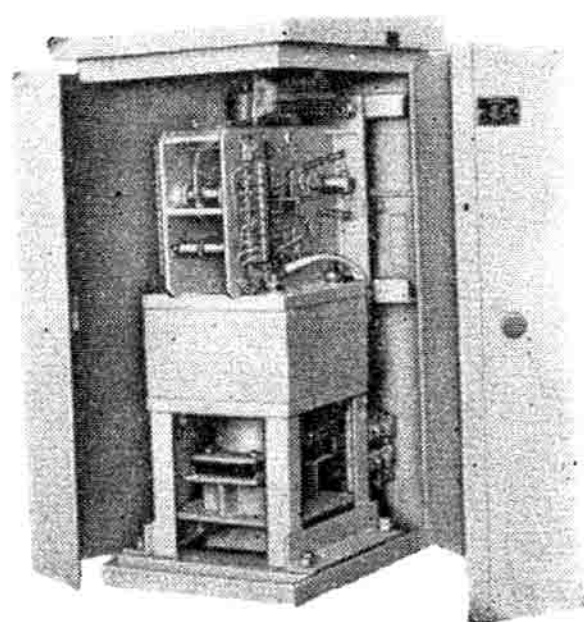
CD3-XG型直流电磁式操动机构
