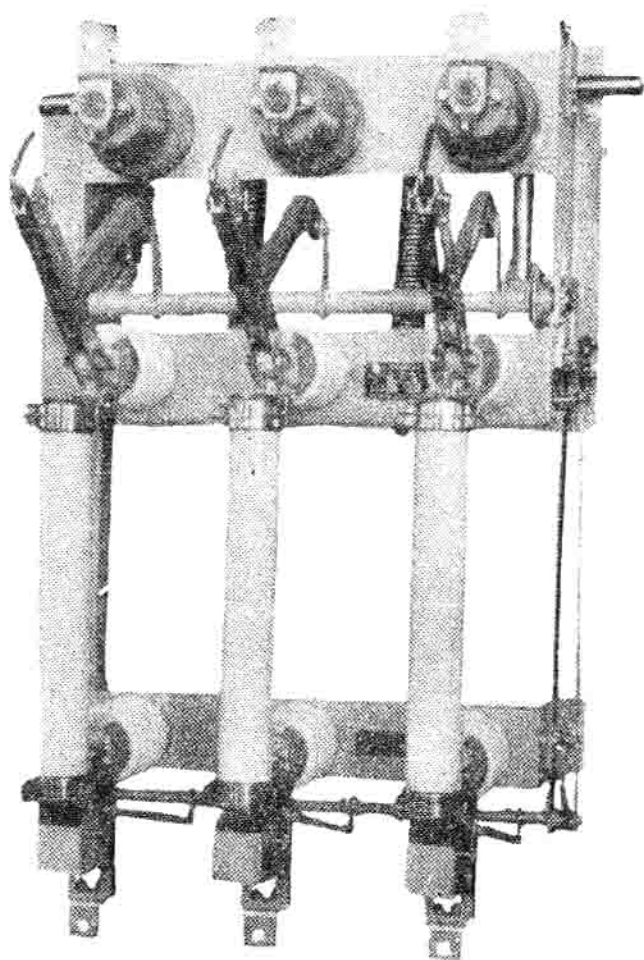
FN3-10户内 压气式高压负荷开关
