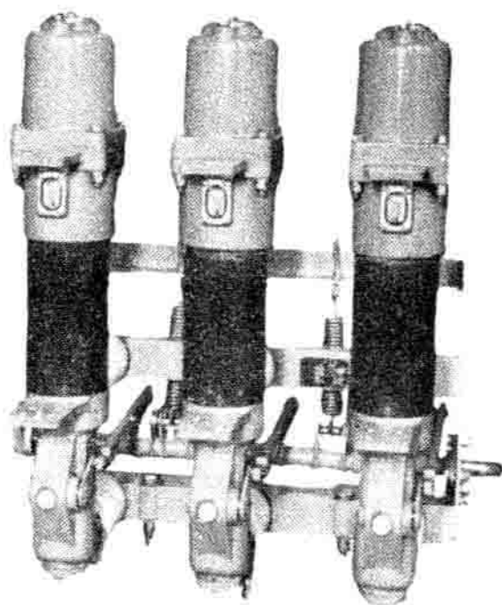
SN10-10 II 型高压户内少油断路器
