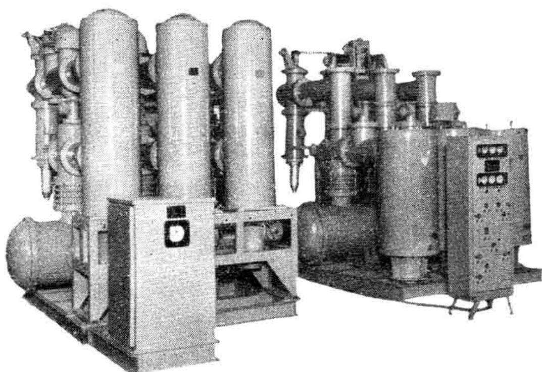
ZF□-110 型六氟化硫全封闭组合电器
