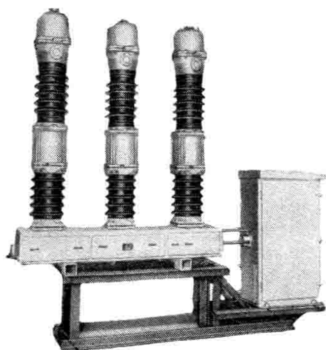
SW2-35户外高压少油断路器
