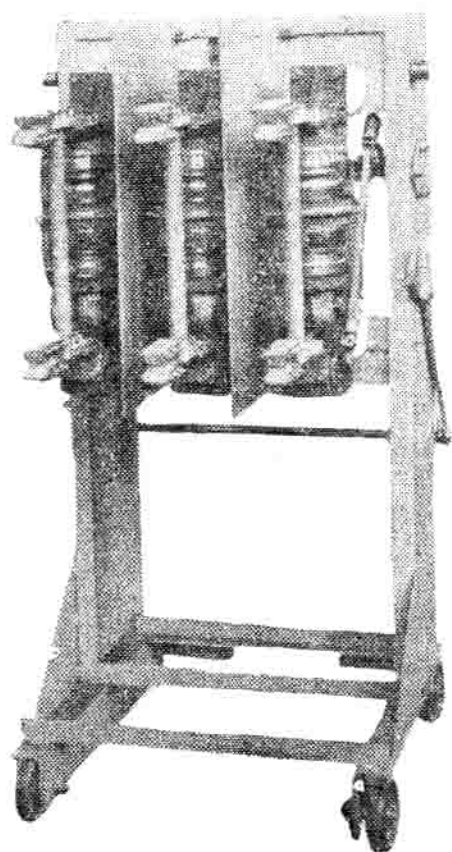
ZN4-10C手车式 高压真空断路器
