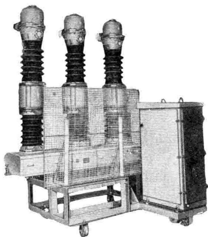
SW2-35C高压手车式少油断路器
