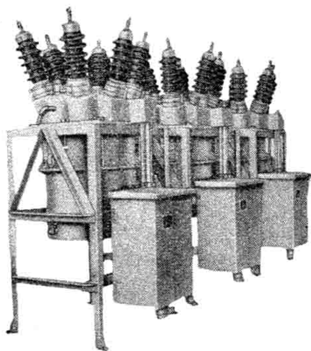
DW6-35 户外 共箱式高压多油断路器
