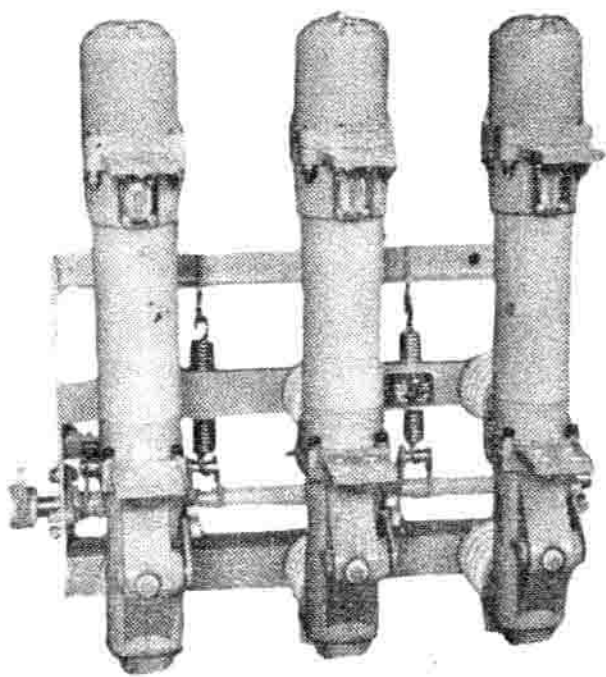
SN10-10 I 型高压户内少油断路器
