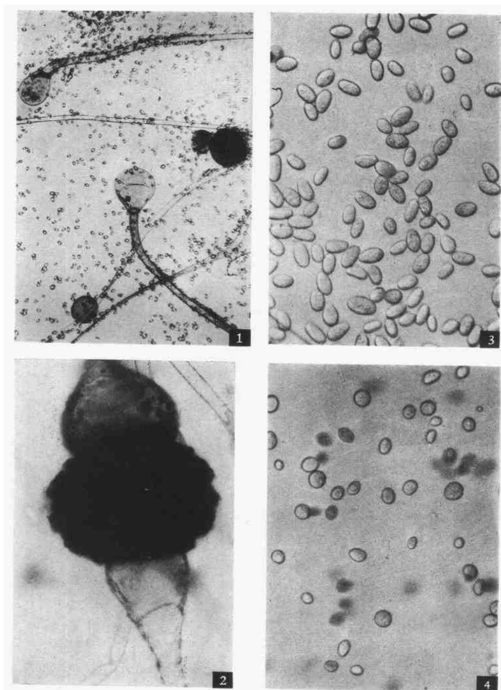
图2 1. G. hainanensis 的孢子囊、孢囊梗和囊轴；2. G. hainanensis 和 G. persicaria 之间形成的接合孢子，两个配囊柄的形态是不同的；3. G. hainanensis 的孢囊孢子；4. G. persicaria 的孢囊孢子。
