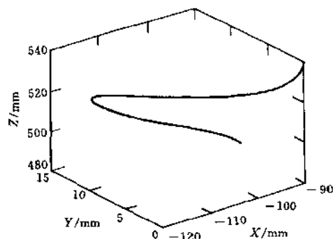
(a) 指端运动轨迹
