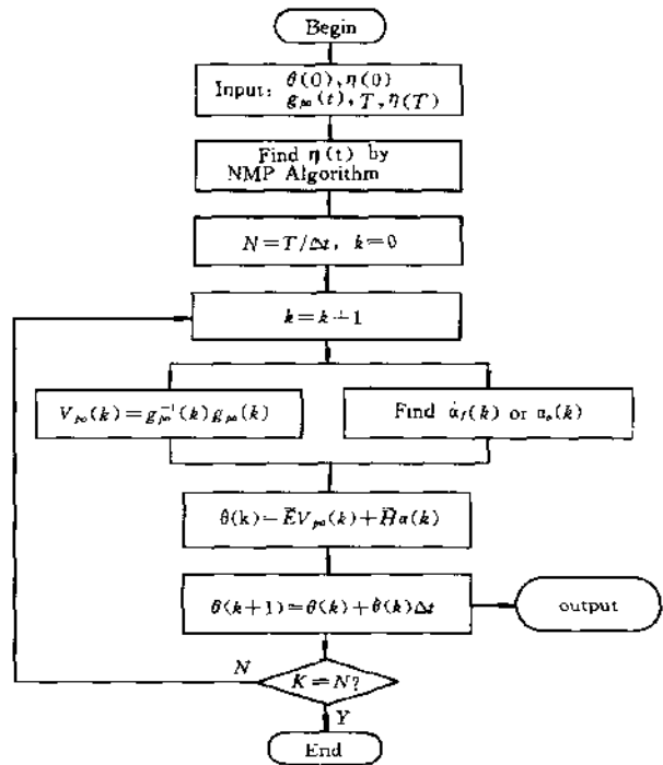
图4 算法过程框图
