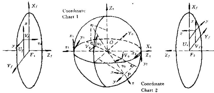
图2 指端和物体的局部坐标系设定
