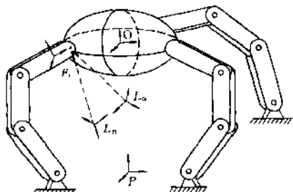
图1 多指手及其坐标系设定
