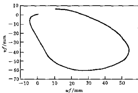
(a) 接触点在指端上的轨迹
