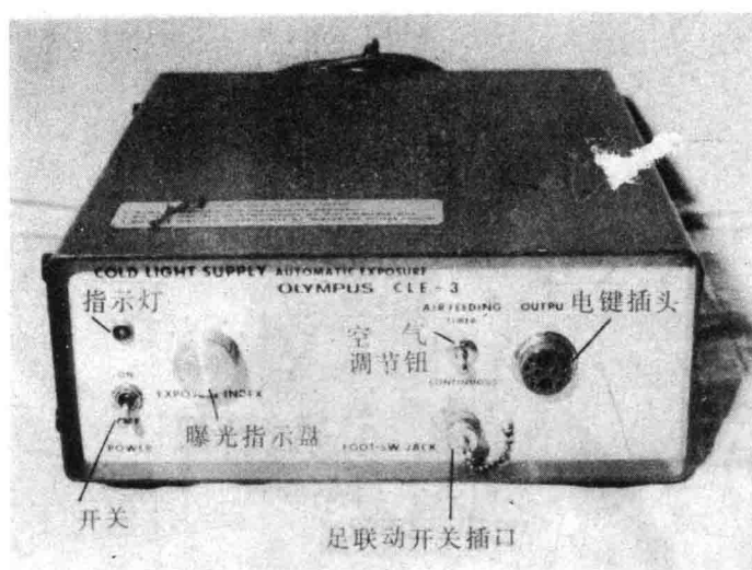
图24-5 冷光源机
