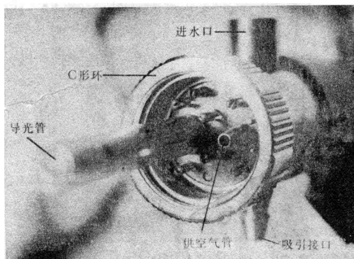
图24 - 4 光源连接部 (放大)
