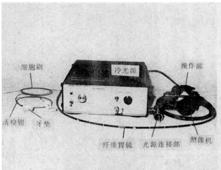
图 24 - 1 一套完整的纤维胃镜
