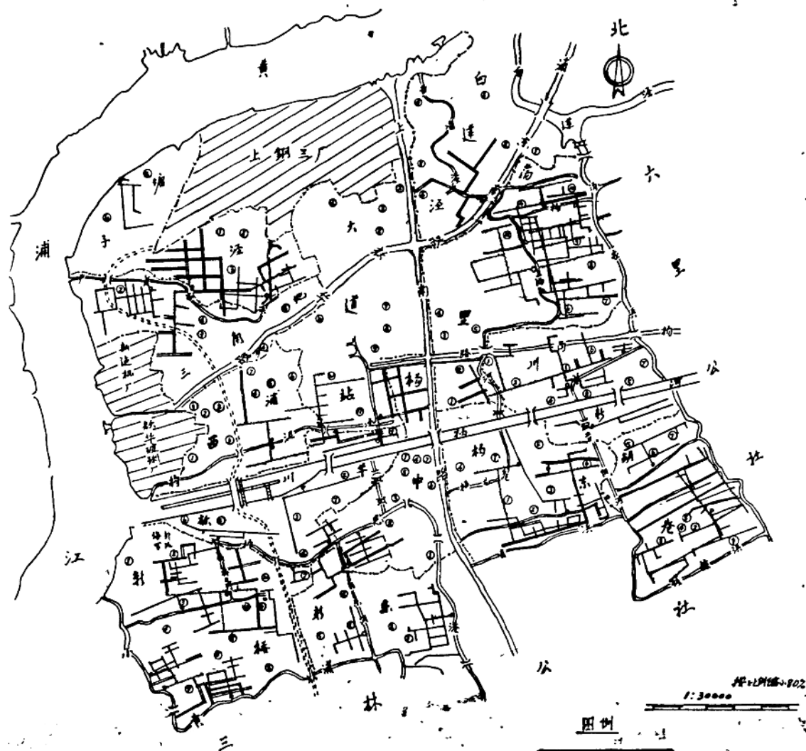
柳巷公社各生产队农田机电灌溉设施图 柳巷公社各生产队农田机电灌溉设施图
