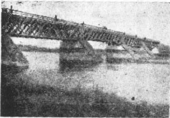
圖6 常用橋型橋(高水位橋)
