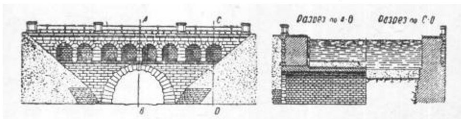
圖14 載水橋
