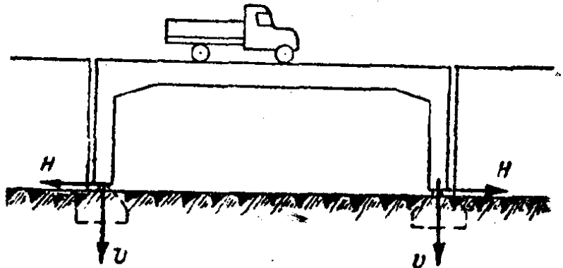
圖18 框 架 橋
