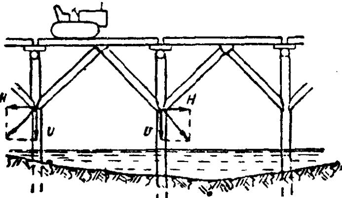
圖17 八字斜撐橋
