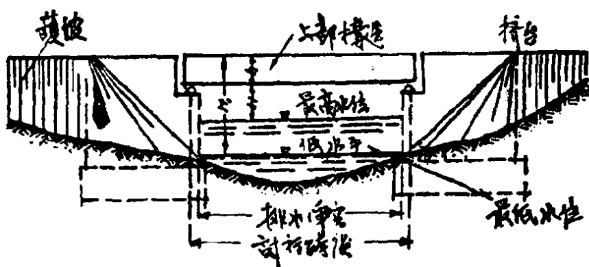
圖 2 單孔橋圖
