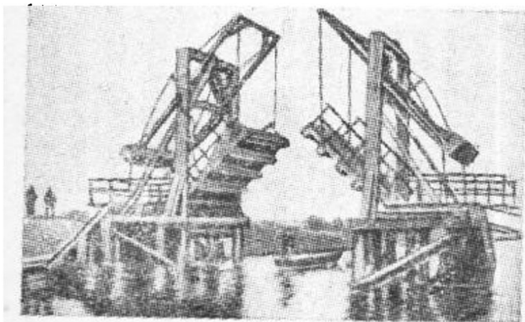
圖 7 開合式橋
