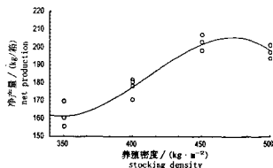
图 1 小网箱养鲤净产量与放养密度的关系
