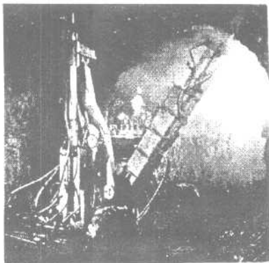
梅山冶金公司铁矿双机掘进台车在作业
