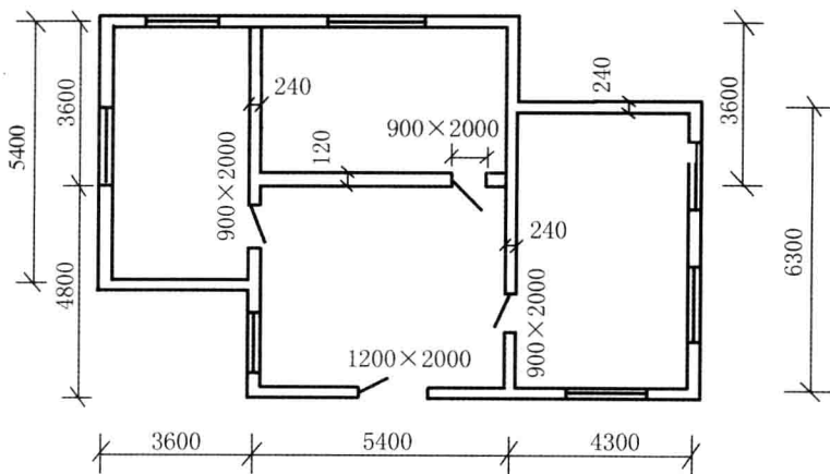
图 1-4 房屋平面示意图
