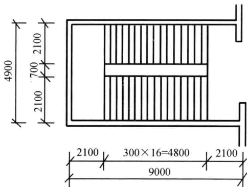
图 1-11 楼梯平面图
