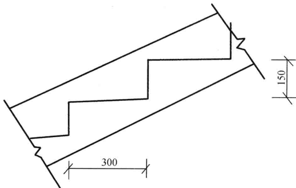
图 1-10 楼梯大样图
