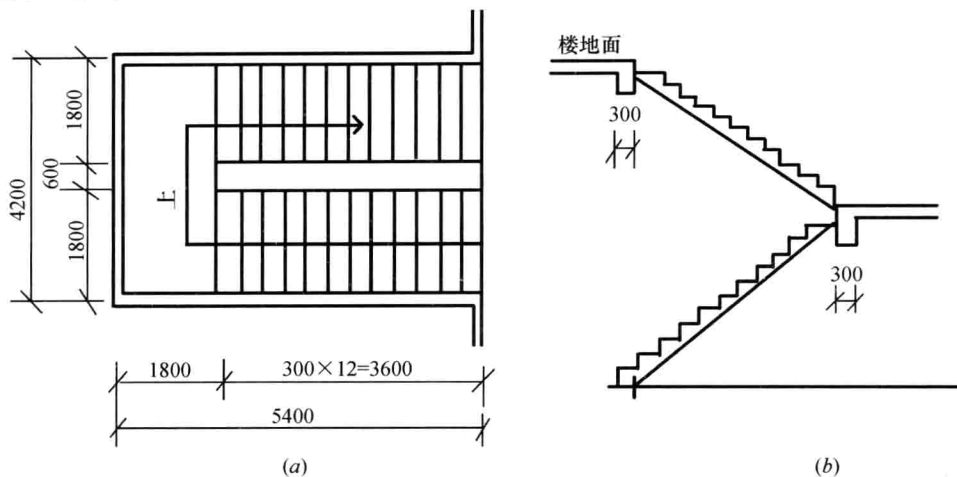
图 1-12 楼梯平、立面图
