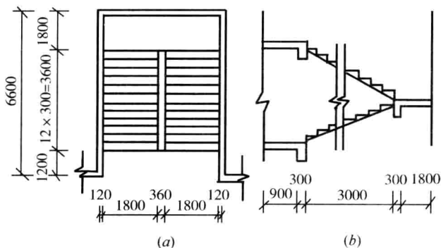
图 1-5 楼梯示意图
