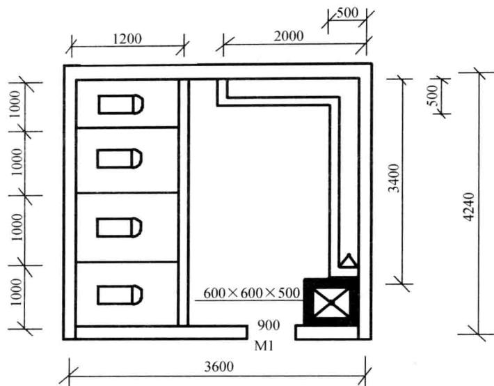
图 1-8 卫生间平面示意图
