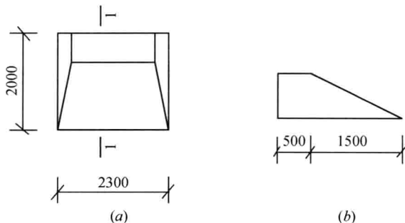
图 1-3 坡道示意图
