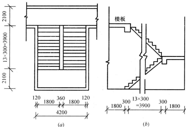
图 1-6 楼梯平、立面示意图
