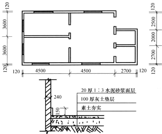
图 1-1 室内整体楼地面示意图
