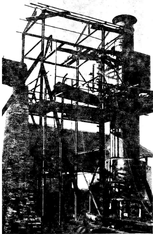
长治附城兵工厂的化铁炉
