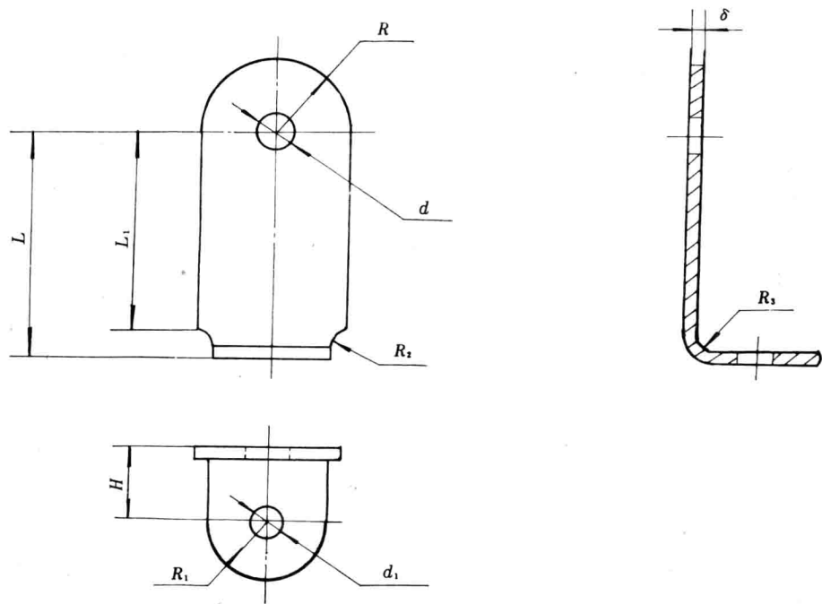
图 1 SP11、SP12 散热器
