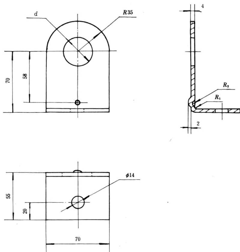
图 5 SL20、SL21 散热器的导电片
