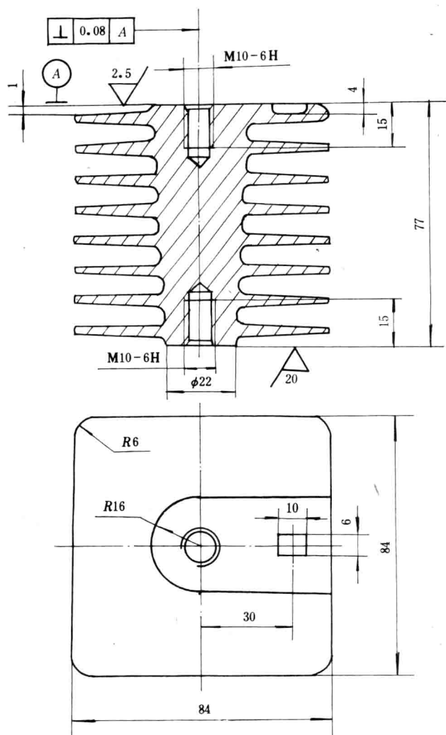
图 7 SZ17 散热器的散热体
