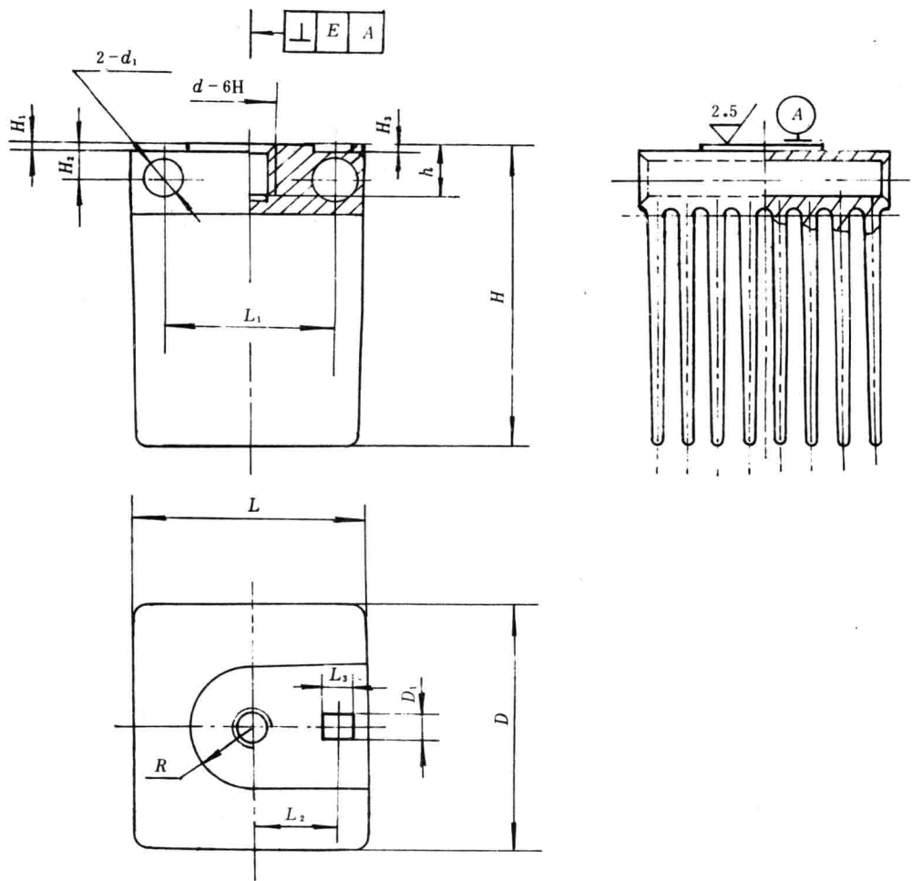
图 8 SL17、SL17B、SL18 及 SL18B 散热器的散热体 表 8
