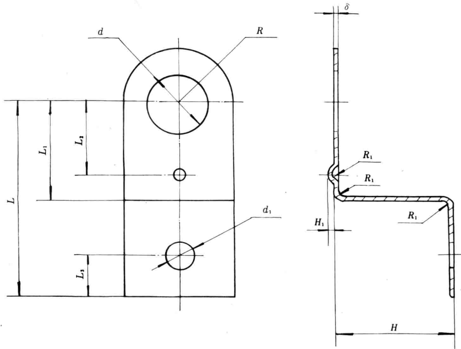
图 4 SL17、SL17A、SL18、SL18A、SL19、SL19A 散热器的导电片
