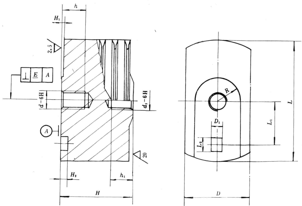
图 6 SZ13、SZ14、SZ14A、SZ14B、SZ15、SZ15A、SZ16 及 SL16 散热器的散热体
