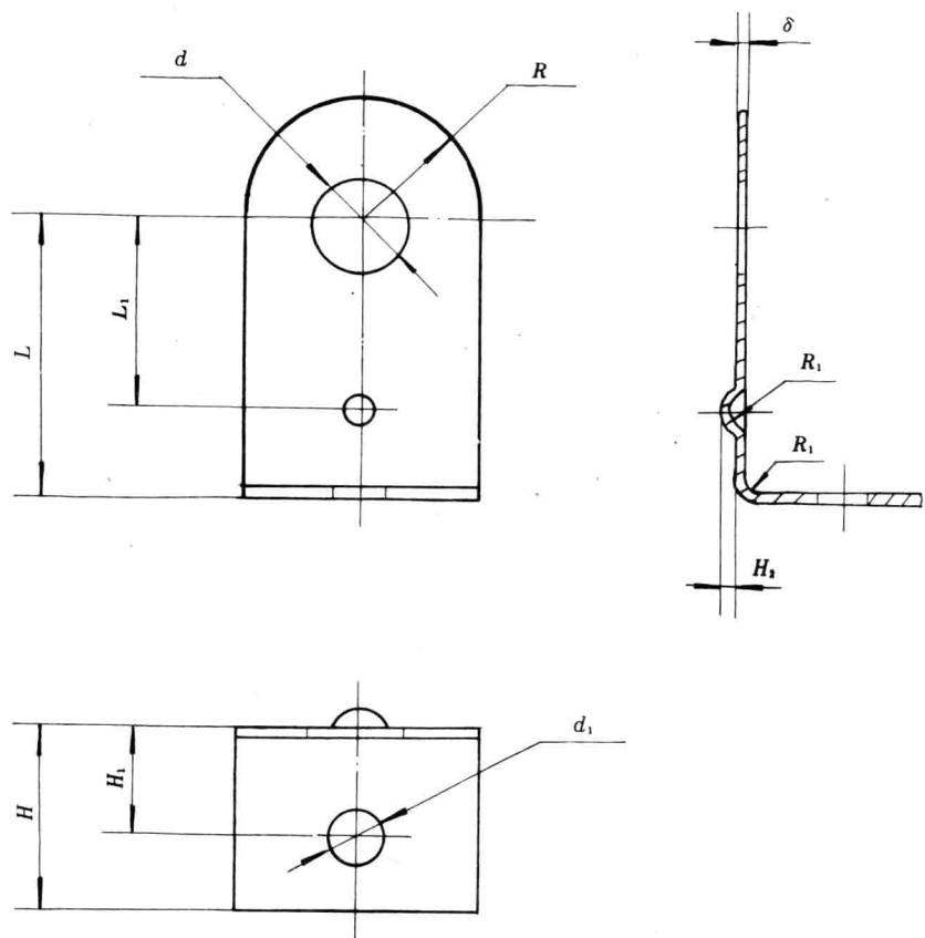
图 3 SZ15、SZ15A、SZ16、SZ17、SL16 散热器的导电片
