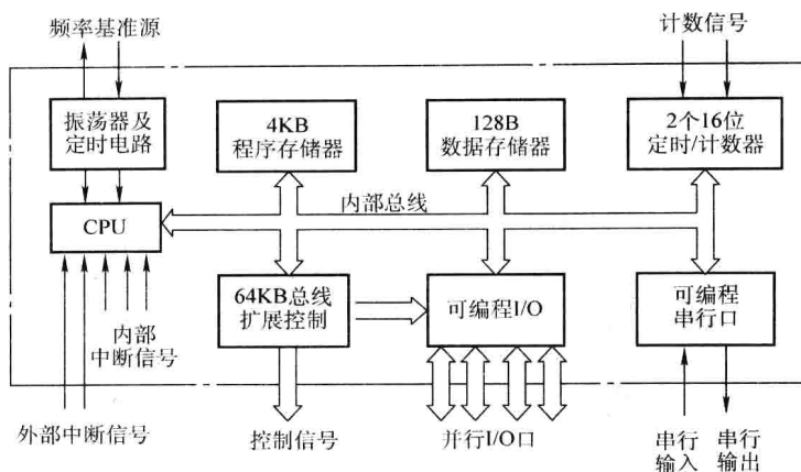
图 2-2 8051 结构框图
