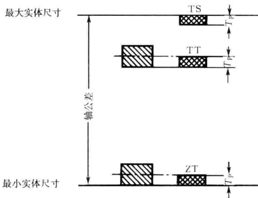
校对量规公差带图
