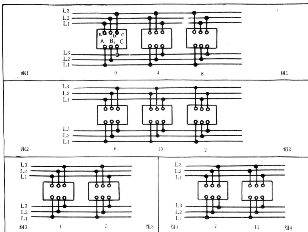
图2 同组变压器的并联运行
