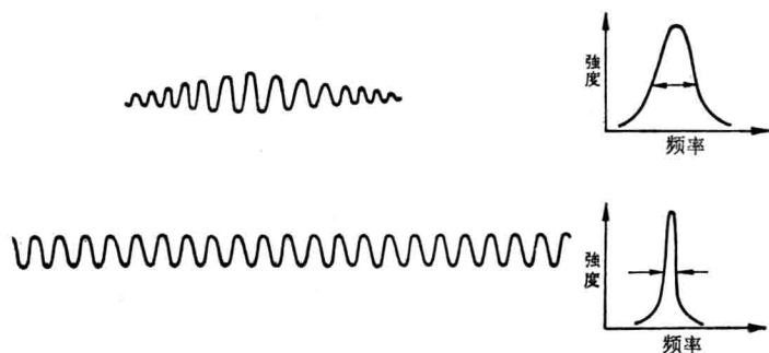
图 1.3 持续时间越长,谱线宽度就越窄
