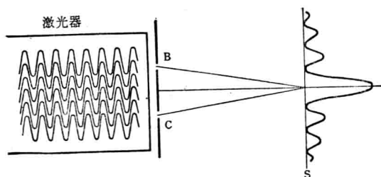
图 1.8 激光束的干涉实验
