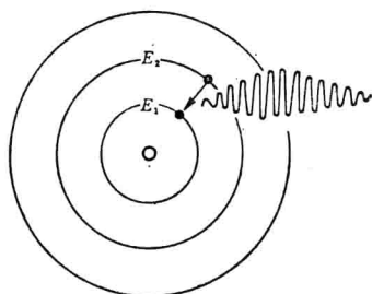
图 1.1 电子从能量 E_2 跃迁至 E_1 态时, 发射频率 \nu = \frac{E_2 - E_1}{h} 的光子。 h 是普朗克常数, h = 6.6256 \times 10^{-27} 尔格·秒 构成光源的各原子在相互独立的任意时刻发射这样一段一段的光波, 所以即使它们的频率都相同, 彼此的相位也完全无关(图 1.2)。
