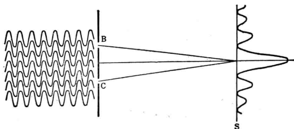
图 1.6 从光源的空间上不同的两点发出相位一致的光, 则穿过两个缝隙后将在屏 S 上产生干涉条纹
