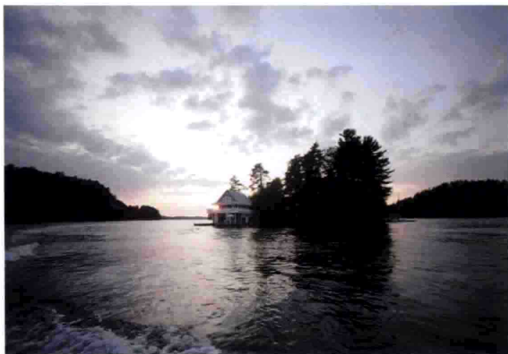
湍流的中心
