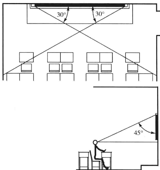
图 1.7 教室座位的视角
