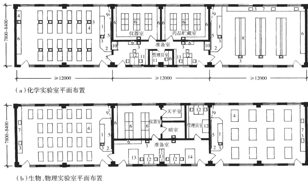
(b) 生物、物理实验室平面布置
