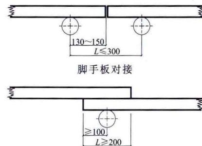
脚手板搭接
