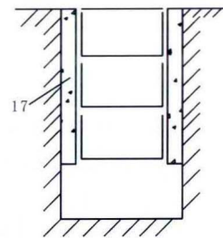
钢筋混凝土支护
