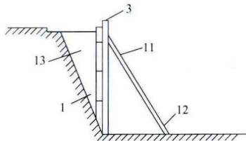
斜柱支撑
