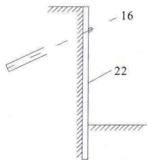
地下连续墙锚杆支护
