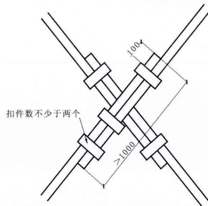
剪刀撑节点放大图
