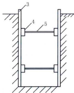
连续式垂直支撑
