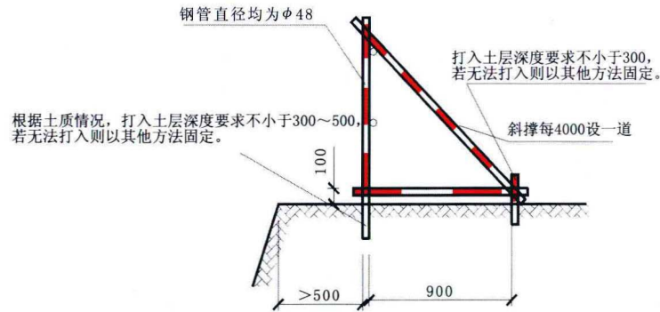
基坑临边防护栏杆局部放大示意图
