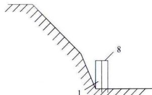
短柱横隔支撑
