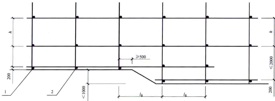
1-横向扫地杆；2-纵向扫地杆
