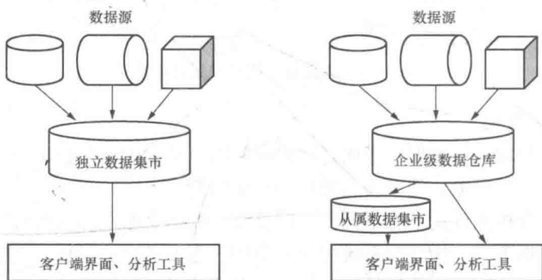
图 1-5 独立型数据集市和从属型数据集市的逻辑结构
