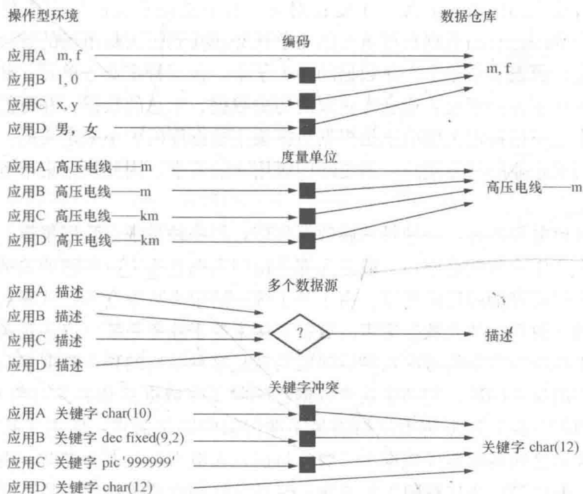
图 1-3 数据由面向应用的操作型环境向数据仓库传送时所进行的集成
