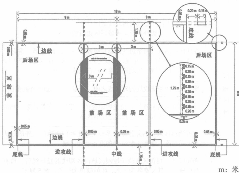
图 4 排球场地画线示意图
