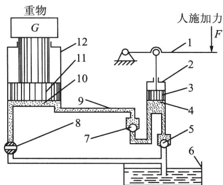
1—杠杆; 2—泵体; 3、11—活塞; 4、10—油腔; 5、7—单向阀; 6—油箱; 8—放油阀; 9—油管; 12—缸体
