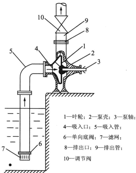
图 1-2 离心泵的工作原理
