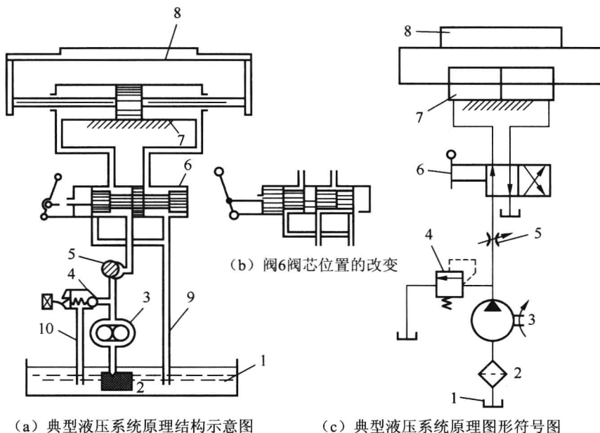
1—油箱；2—过滤器；3—液压泵；4—溢流阀；5—流量控制阀； 6—换向阀；7—液压缸；8—工作台；9、10—管道
