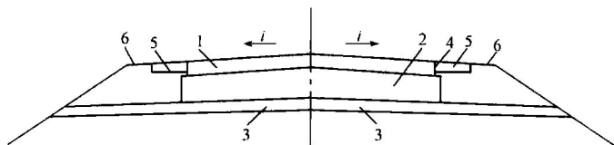
图 1-2 路面结构层次划分示意图
