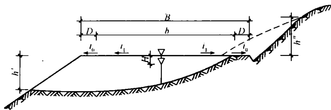
图 1-1 路基基本构造图
