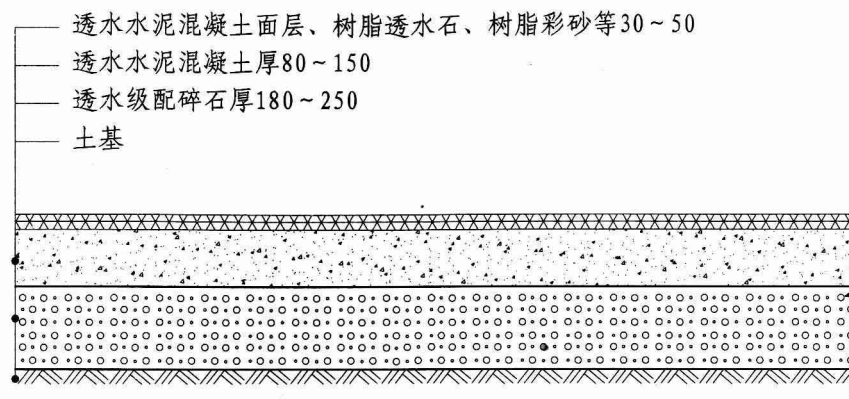
无停车透水水泥混凝土基层人行道结构图(三)
