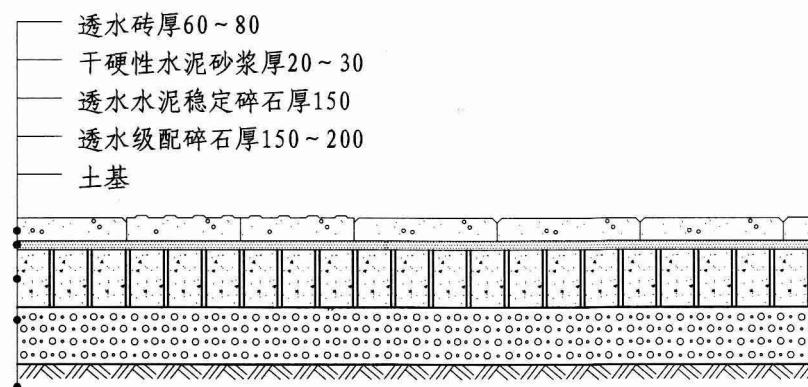
无停车透水水泥稳定碎石基层人行道结构图（二）
