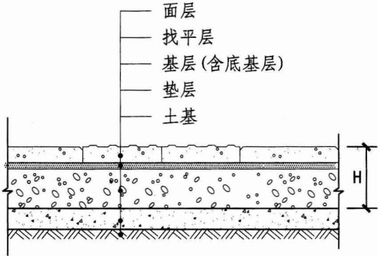
透水人行道基本结构组合图
