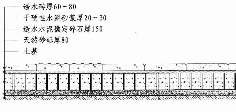
无停车透水水泥稳定碎石基层人行道结构图（一）
