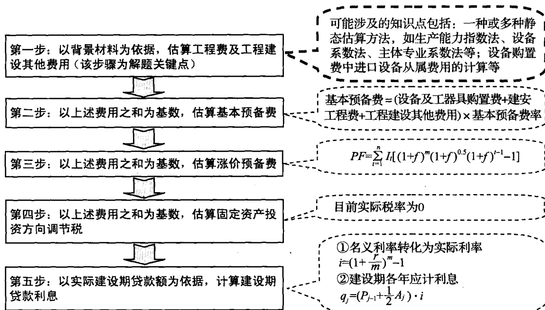
图 1-2 建设投资估算解题步骤
