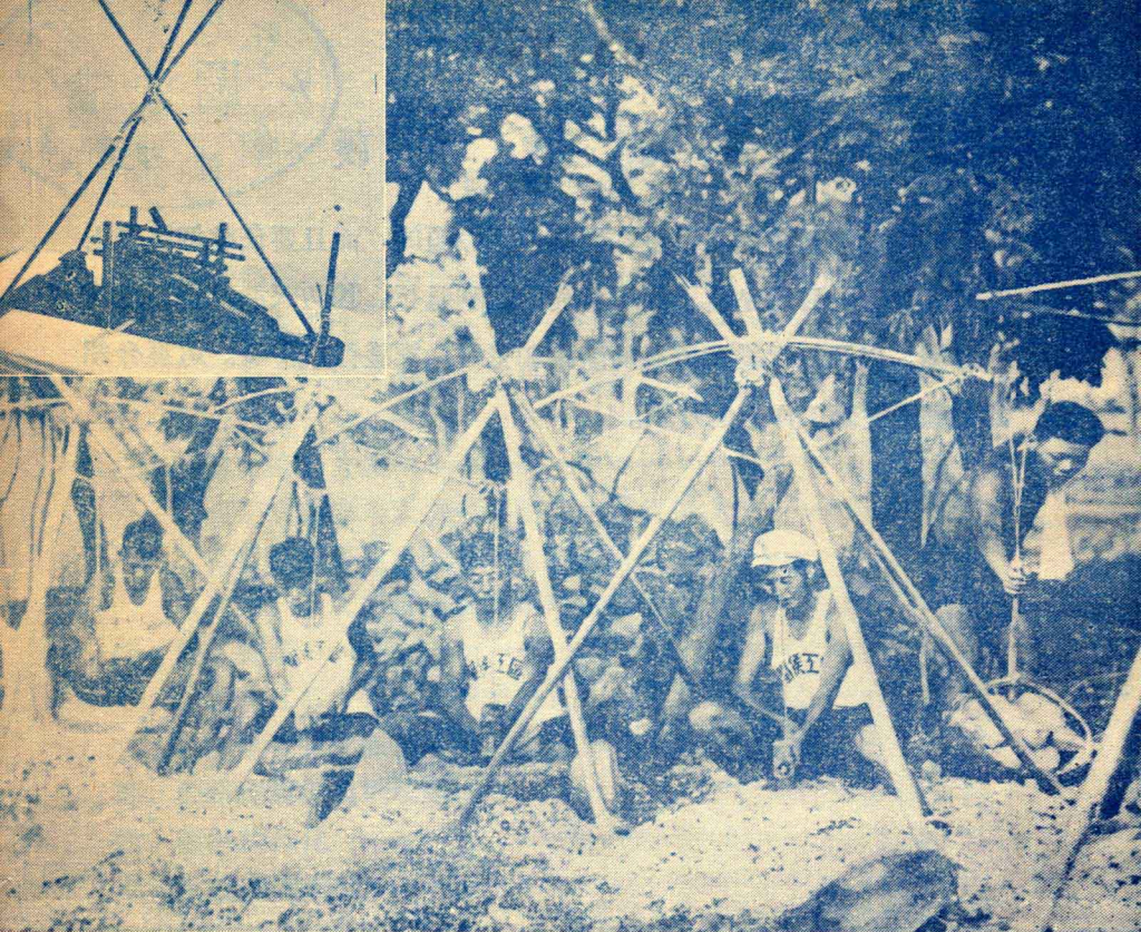
1.準備經常養護道路的碎石，用月弓敲石法敲打碎石。左上圖為「三弓敲石推篩機」的模型，敲篩同時進行，工效可達 1.1 公方。
