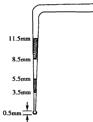
图 1-1 CPI 探针的探头
