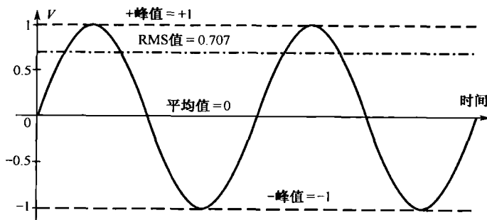
图 1-7 RMS 值和其他测量值的关系
