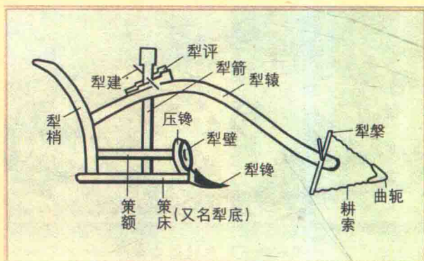
图1-7 曲辕犁
