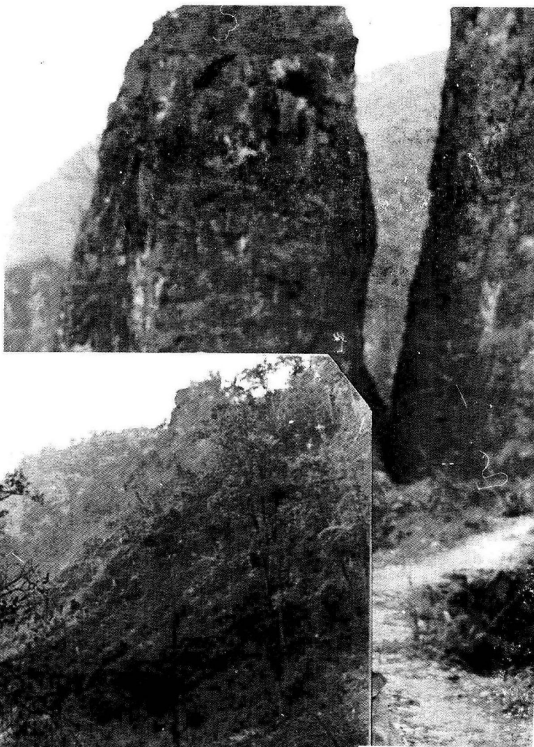
▷ 乌伞冲引水渠道险要渠段(一线天段), 渠长 23 米, 开凿高度 33 米。
