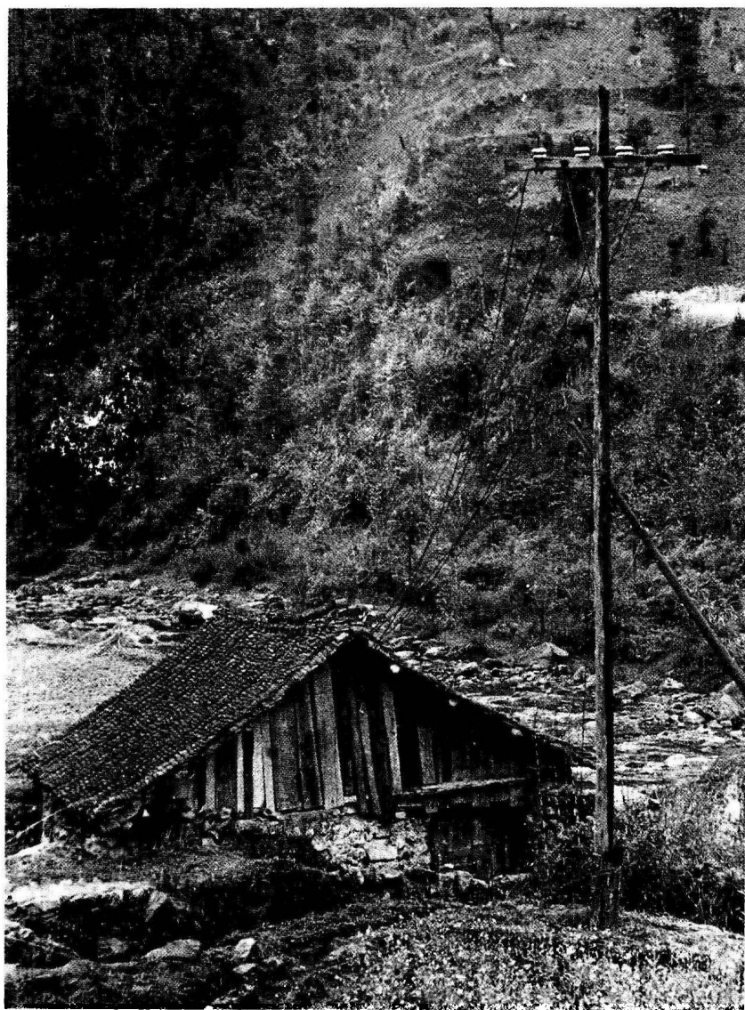
△谷江清塘简易水电站
