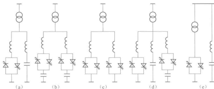
图 1-1 晶闸管控制 SVC 的结构型式
