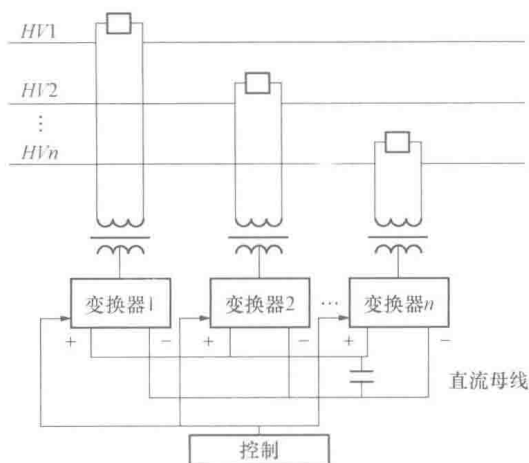
图 1-7 IPFC 基本结构图
