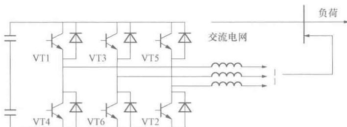
图 1-2 STATCOM 基本结构图
