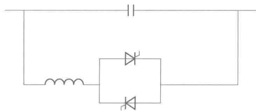
图 1-3 TCSC 基本结构图
