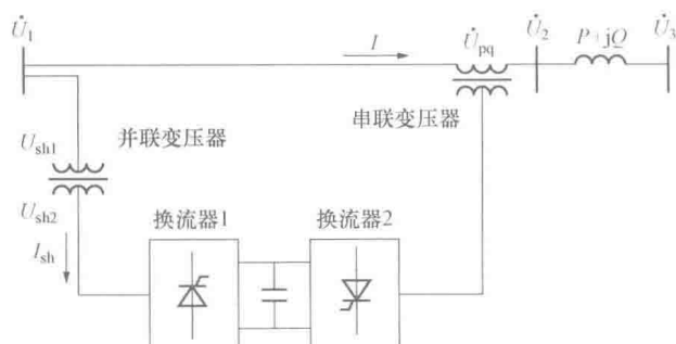
图 1-6 UPFC 基本结构
