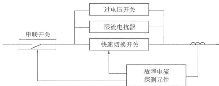
图 1-5 FCL 原理图
