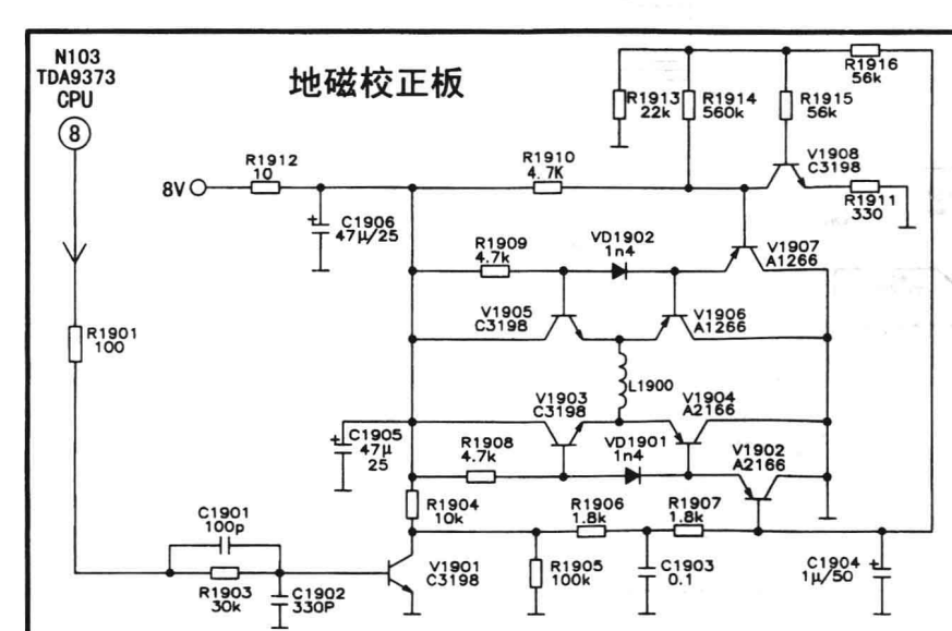
34英寸、29英寸纯平彩管SK型机可设地磁校正板
