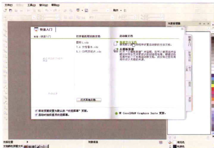
图1-8 欢迎窗口
