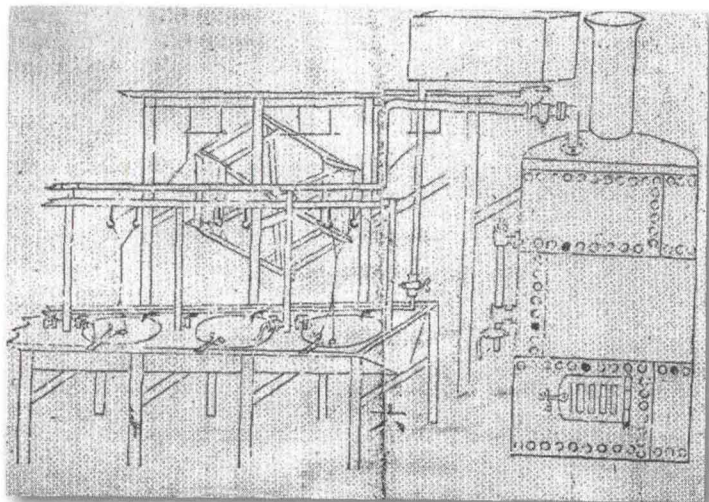
▲ 陈启沅设计的继昌隆缫丝厂蒸汽锅炉和缫丝机
