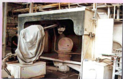
▲ 机械手喷釉(1995年)
