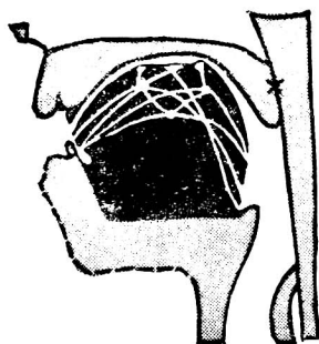
发音部位图
