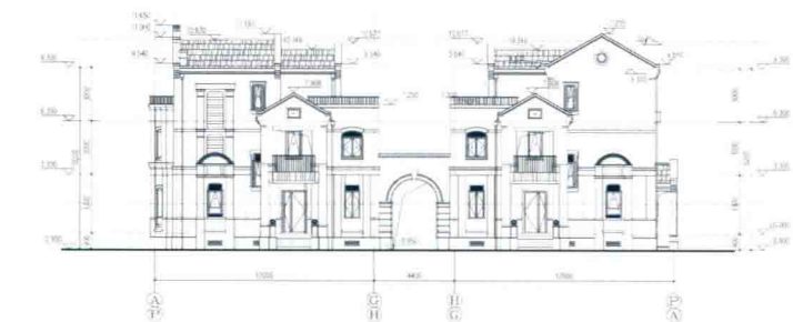
合院轴立面图
