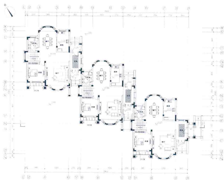
亲水别墅一层平面图
