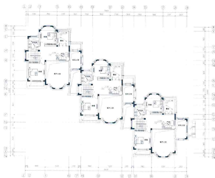
亲水别墅二层平面图
