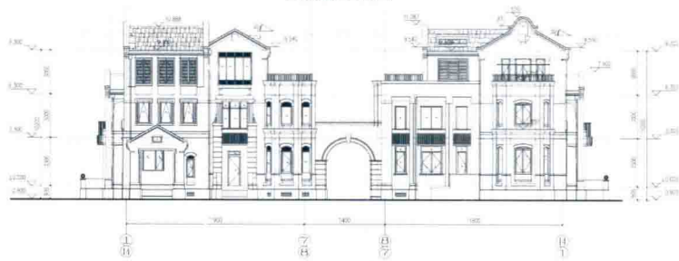
合院轴立面图
