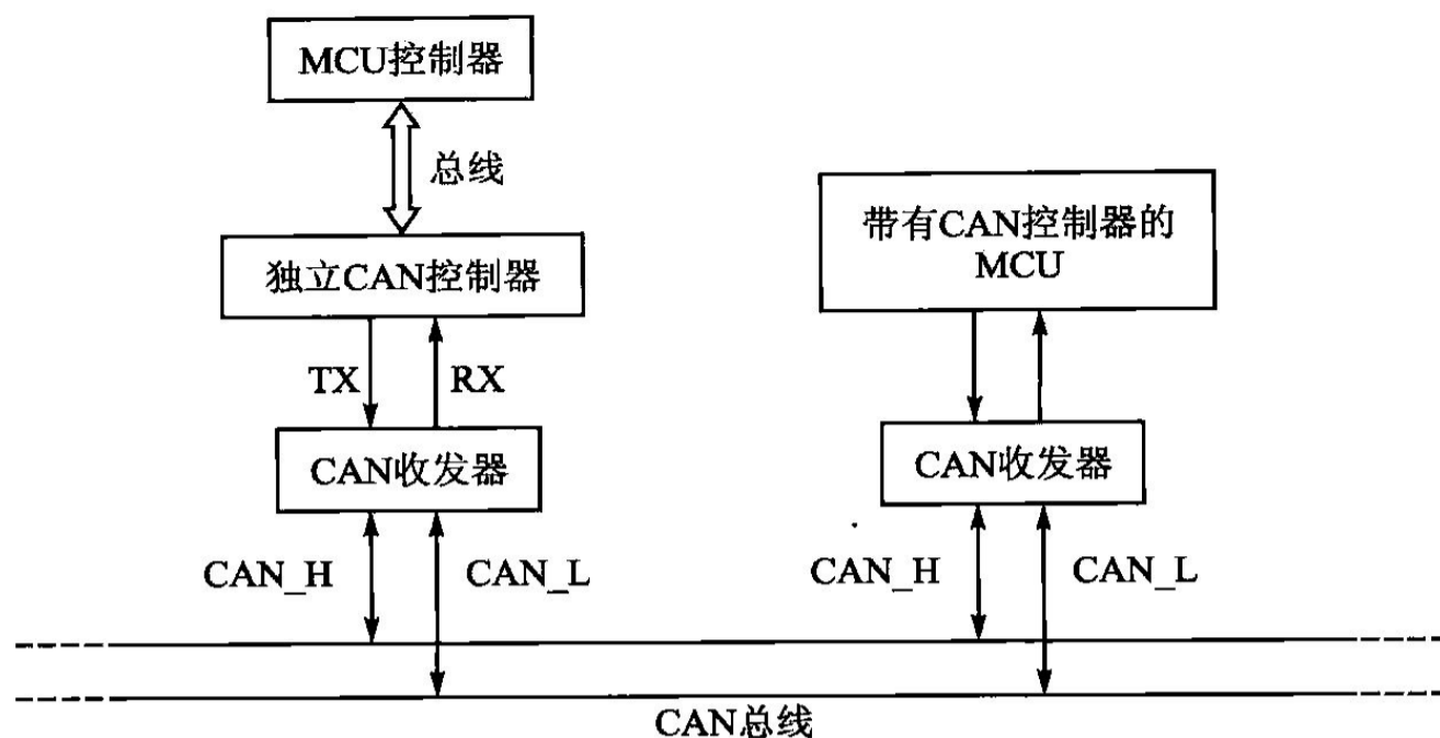
图 1-2 CAN 总线节点的硬件构成
