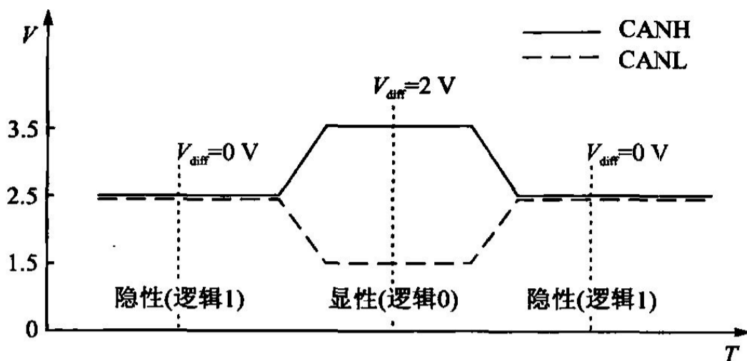
图 1-1 双绞线 CAN 总线电平标称值
