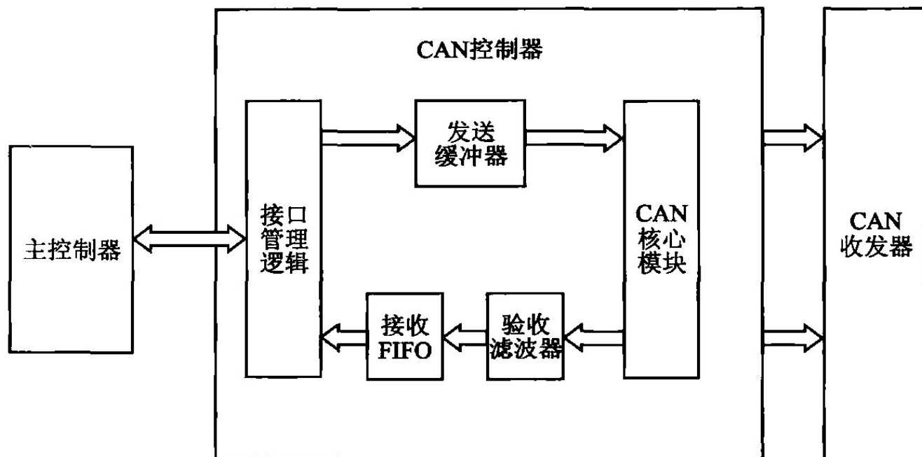
图 1-3 CAN 控制器结构示意图
