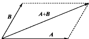
图 1.1.2 平行四边形法则
