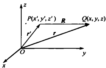
图 1.1.1 距离矢量
