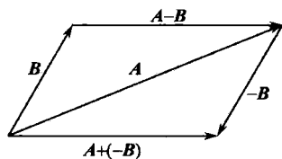
图 1.1.4 矢量求差
