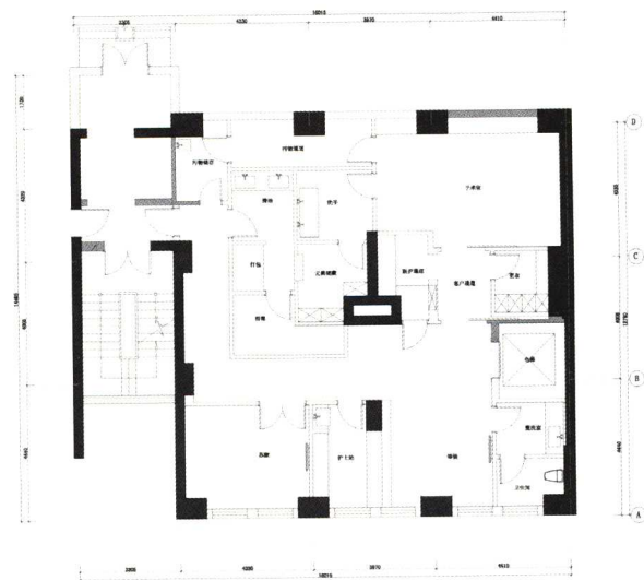
三层平面布置图
